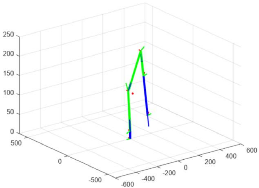
Figura 3.5.13 Geometrie inversă (mișcările robotului la jumătate din iterații)
