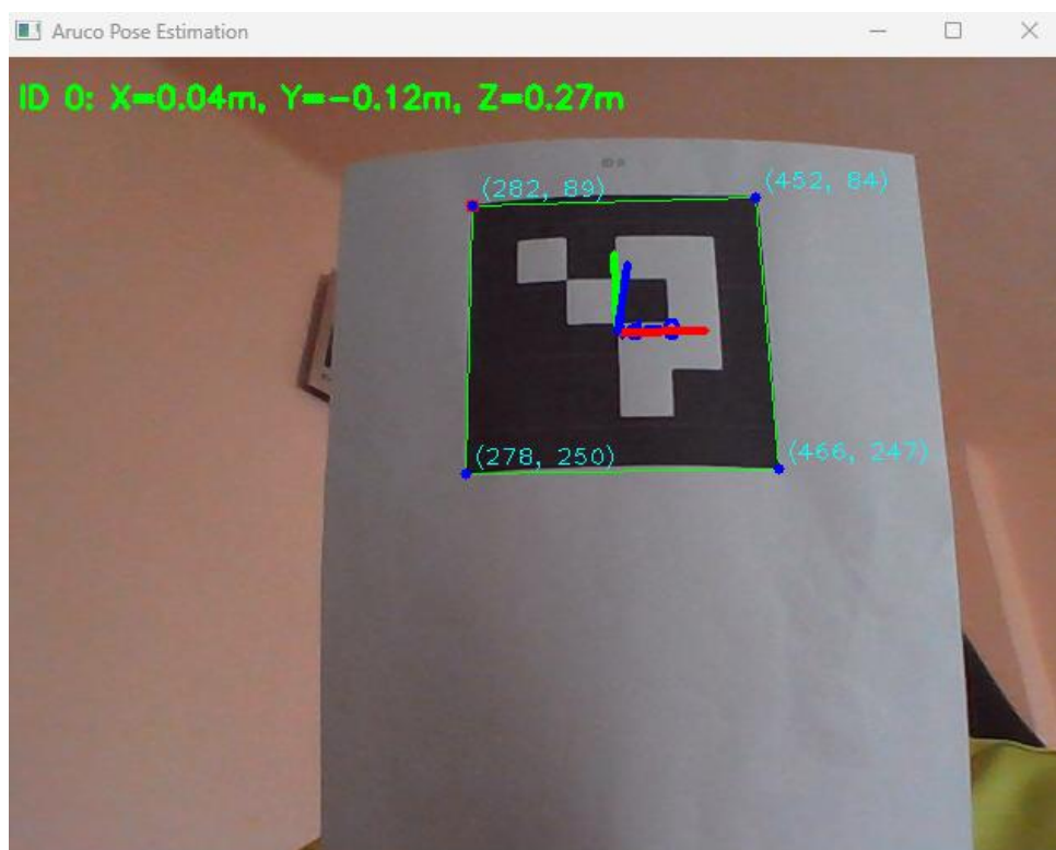
Figura 4.2.1 Cameră calibrate
