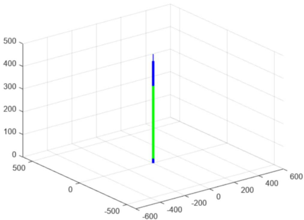
3.5.9 Animație (robotul pleacă de la poziția 0 în toate cuplele și trebuie să se aplice \pi/2 pe cuplele q_3 și q_4 )
