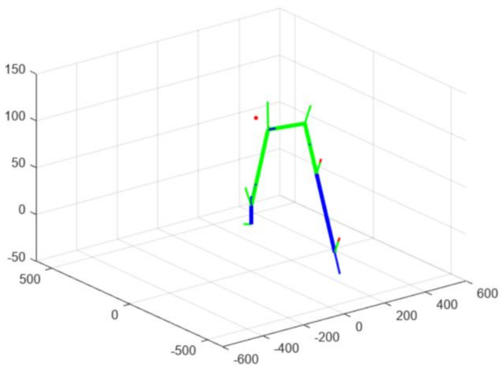
Figura 3.5.12 Geometrie inversă (robotul pleacă de la toate cuplele fiind la \pi/4 și trebuie să ajungă în P_e , adică punctul roșu)
