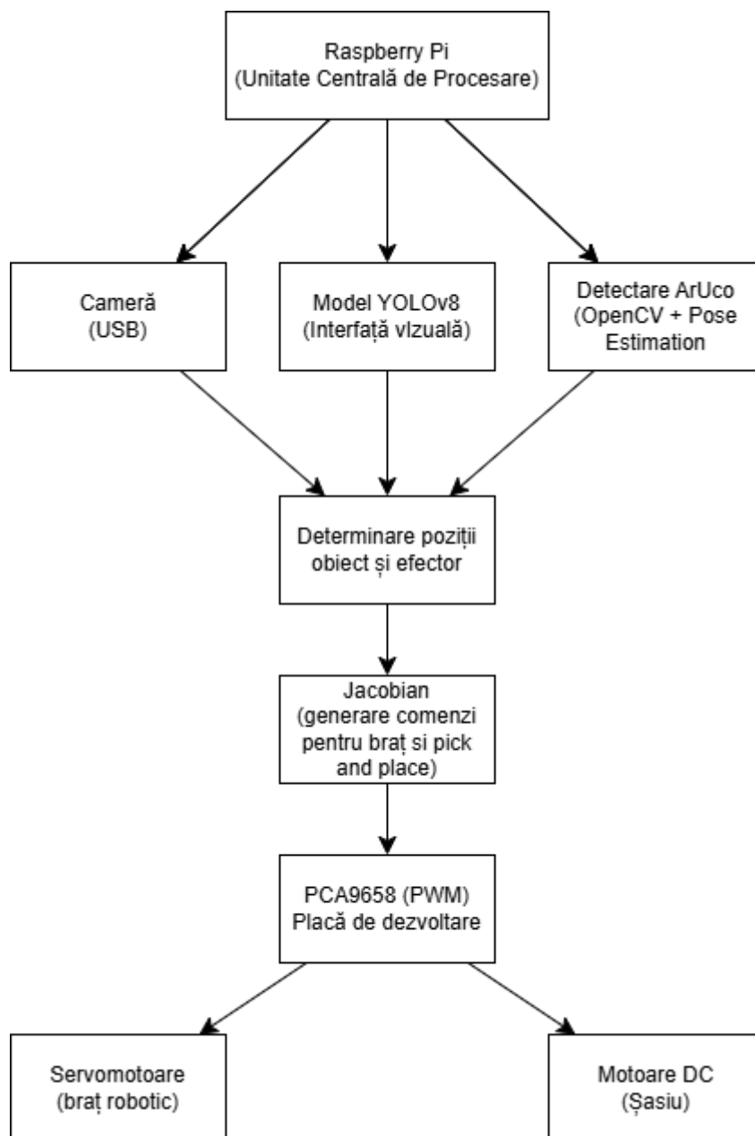
Figura 3.2.1 Diagrama sistemului
