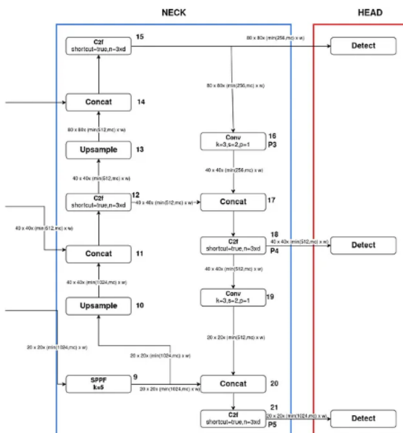
Figura 2.1.3 Neck-ul și Head-ul rețelei [6]
