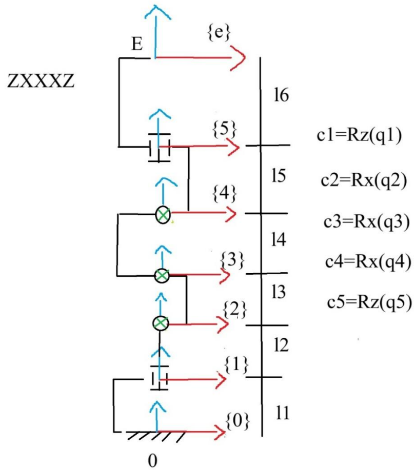
Figura 3.5.1 Desen 5DOF
