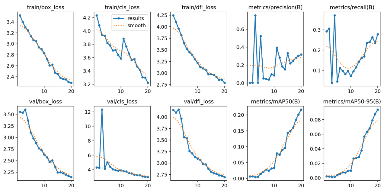
Figura 3.3.3 Rezultate 20 de epoci
