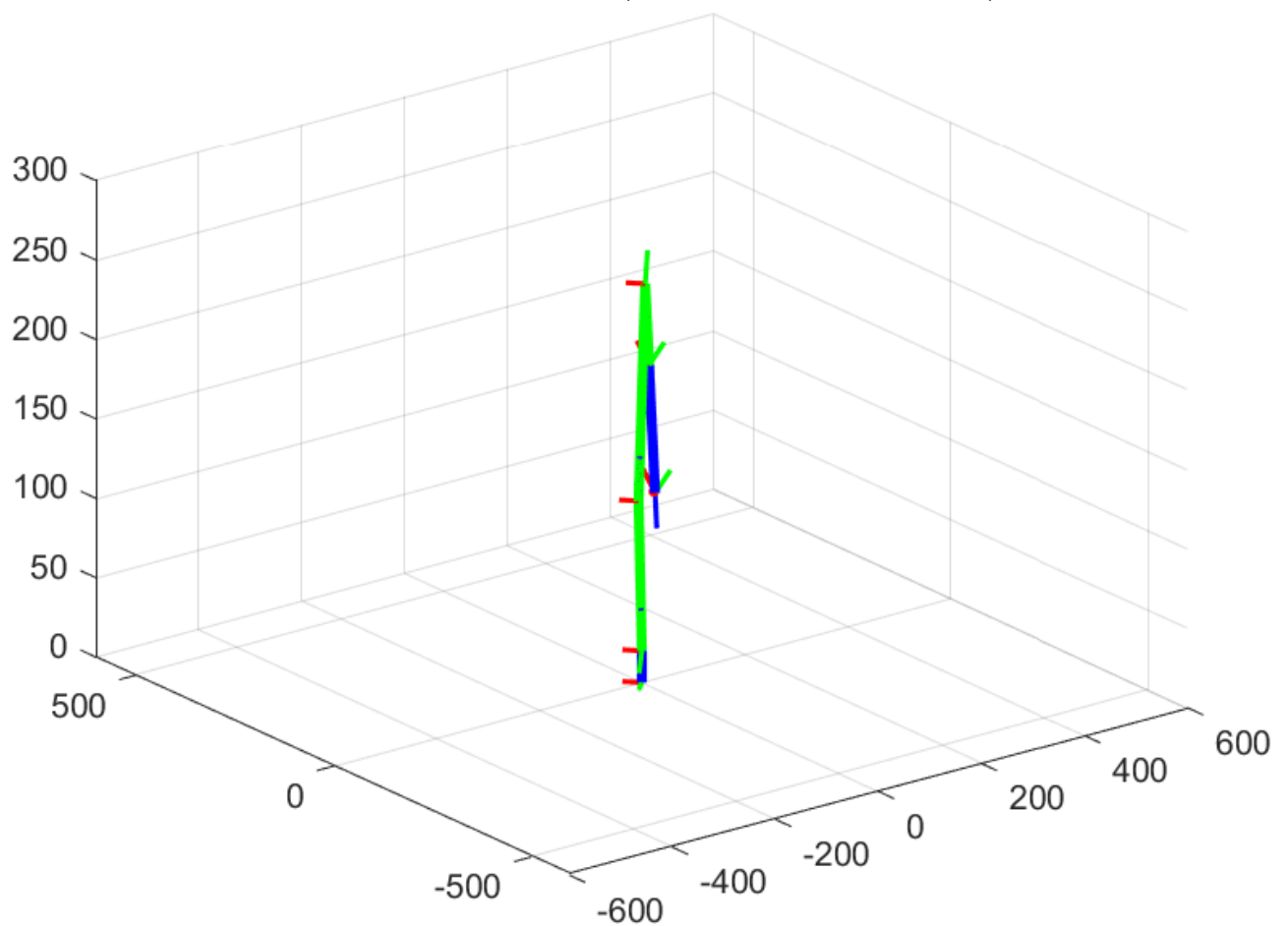
Figura 3.5.14 Geometrie inversă (robotul a ajuns în P_e )
