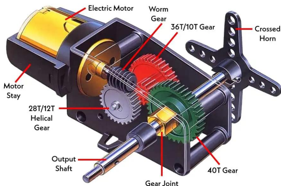
Figura 2.4.1 Construcția unui servo-motor [9]
