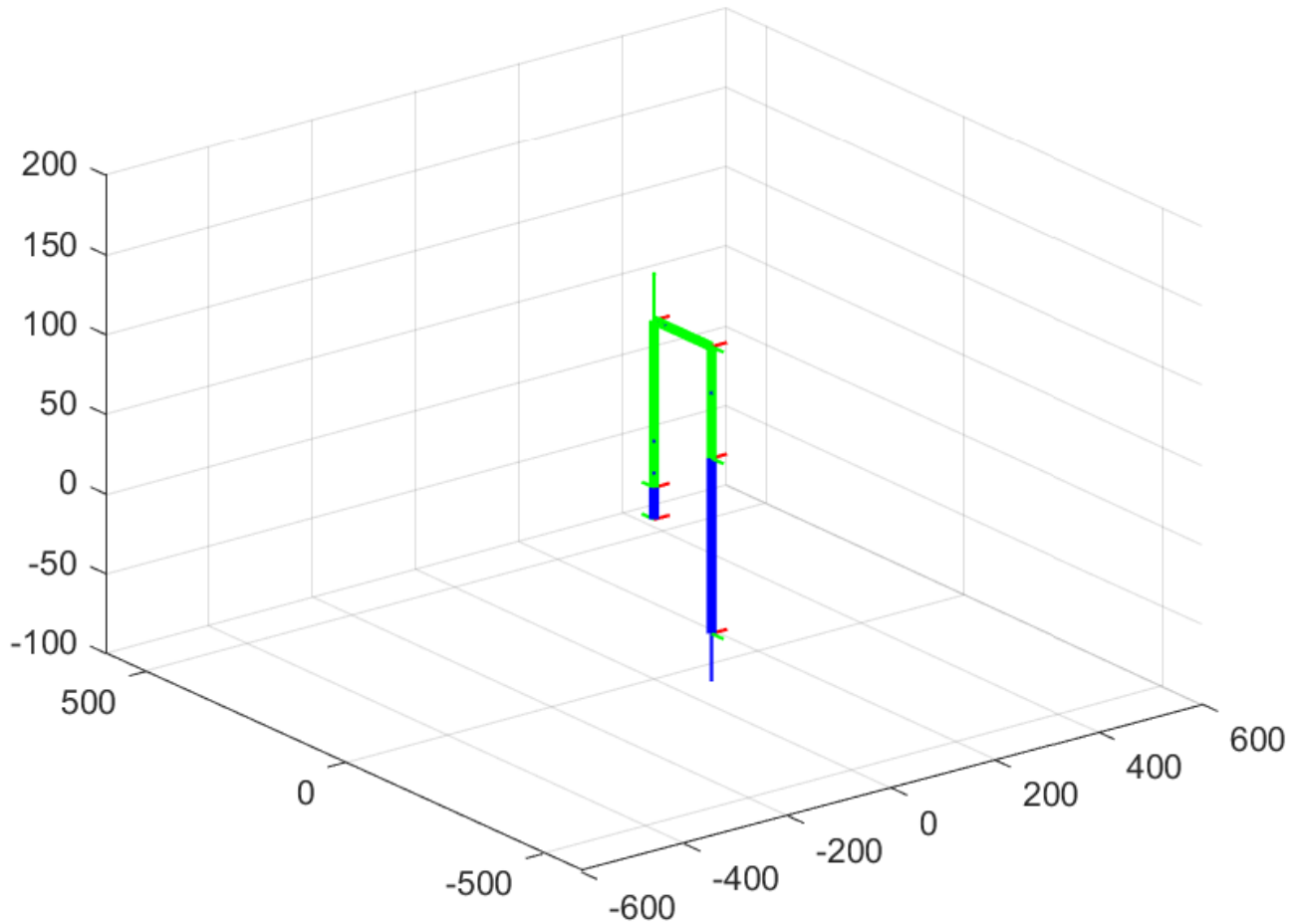
Figura 3.5.11 Animație ( q_4 a ajuns la \pi/2 și robotul s-a mișcat conform impunerii)
