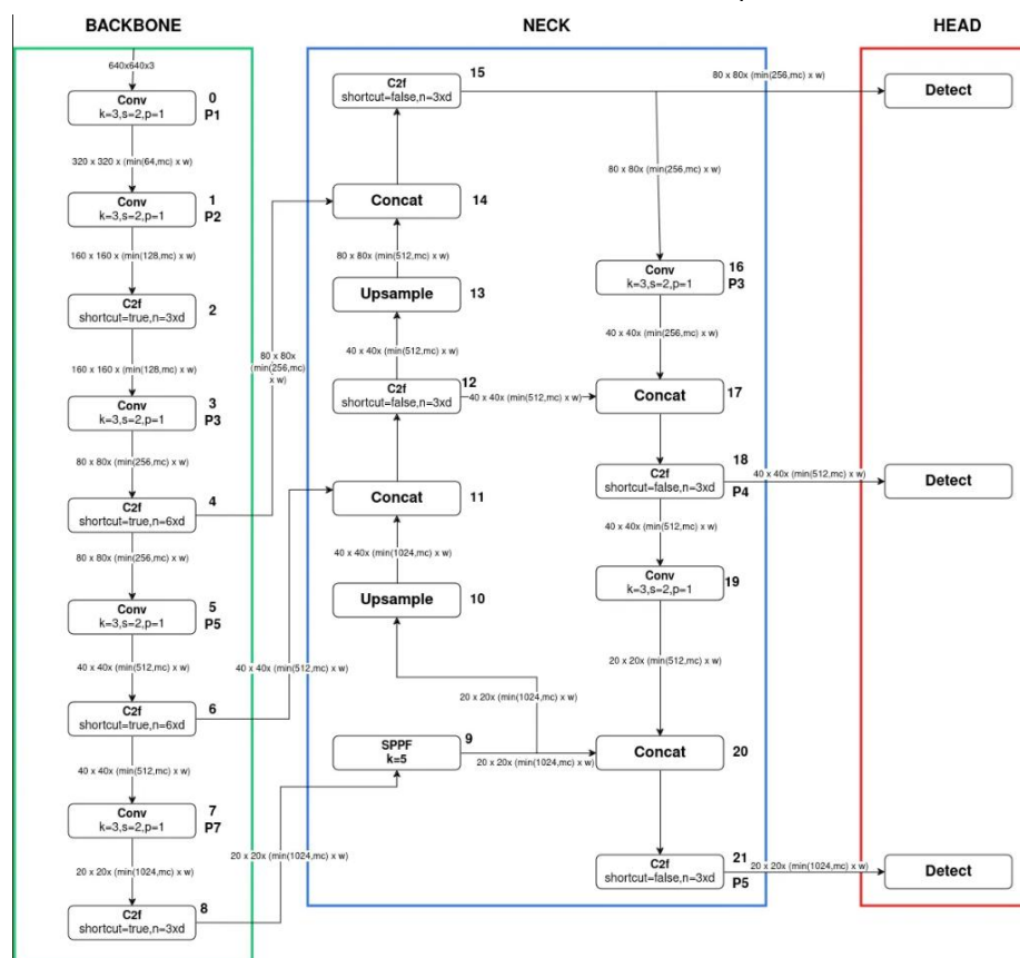
Figura 2.1.1 Arhitectura rețelei de vedere artificială YOLOv8 [6]
