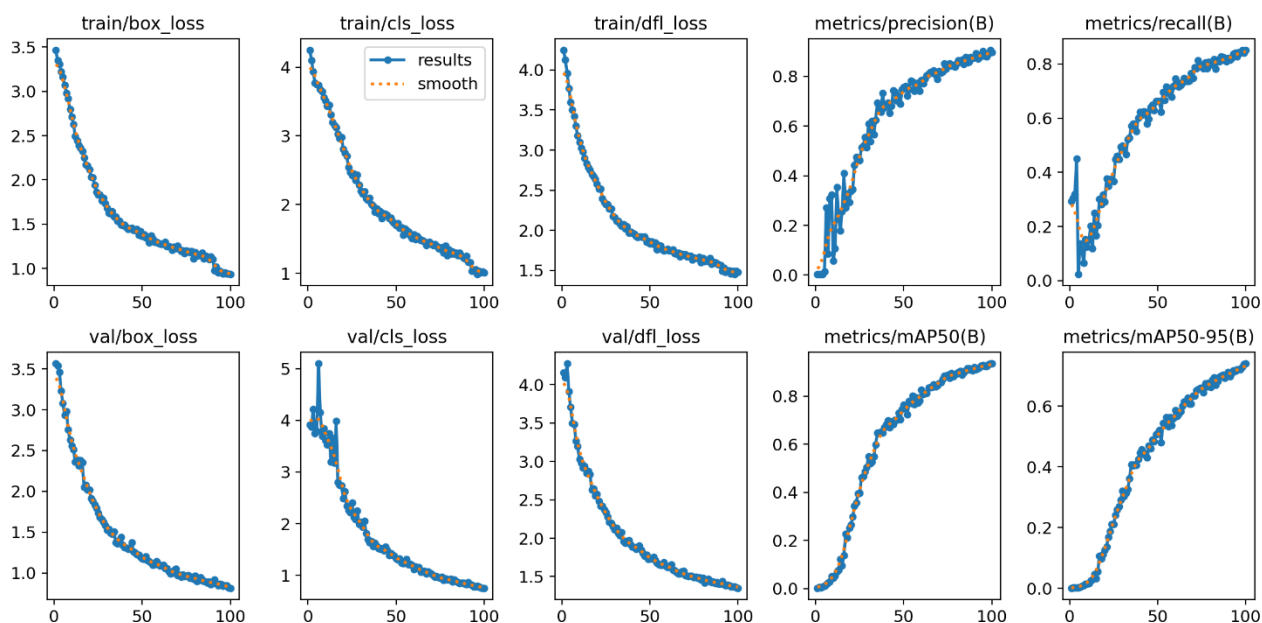
Figura 3.3.4 Rezultate 100 de epoci
