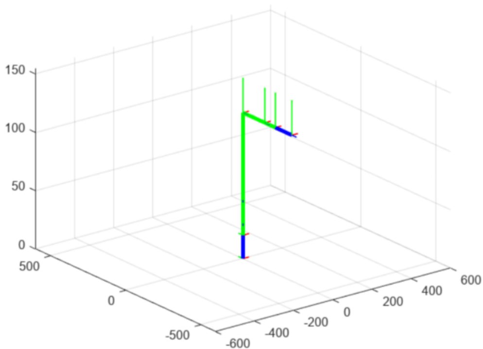
Figura 3.5.10 Animație ( q_3 a ajuns la \pi/2 , iar acum se modifică q_4 )
